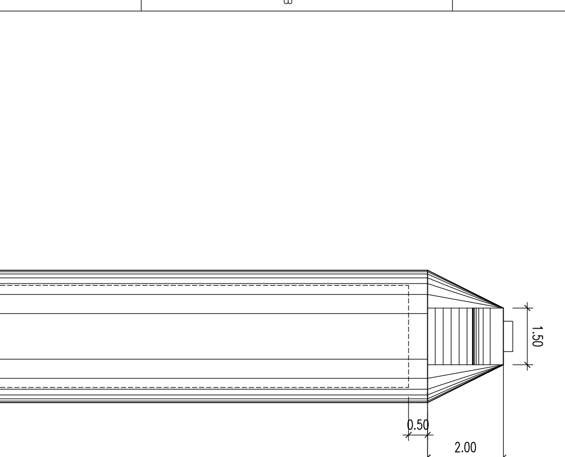
ELEVAZIONE PILI
